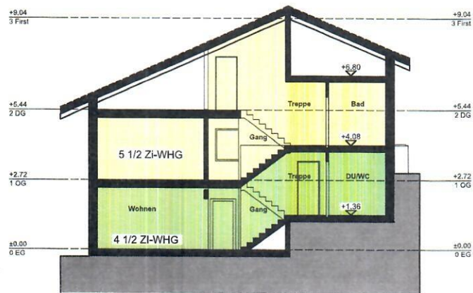
S/01 Schnitt 1:200
