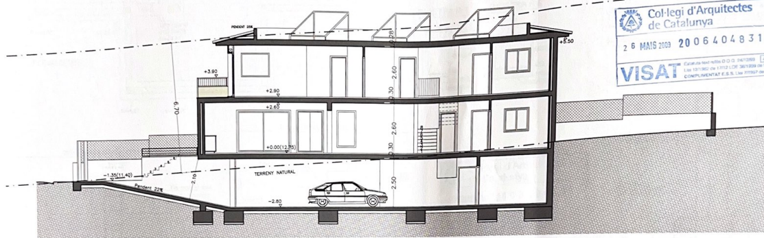
SECCIÓ A-A'
