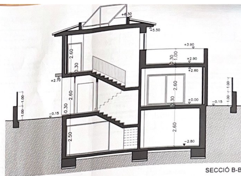
SECCIÓ B-B'
