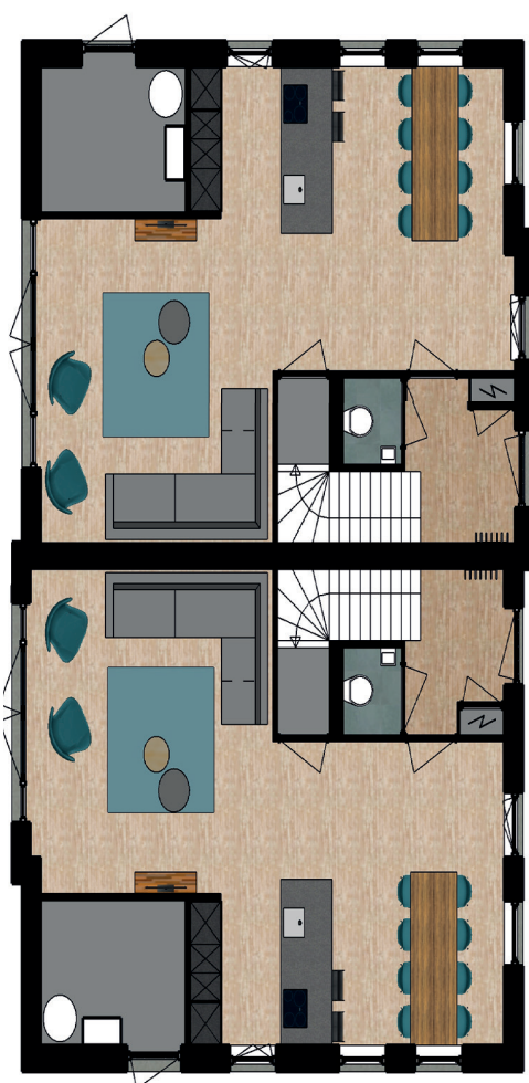
Begane grond
